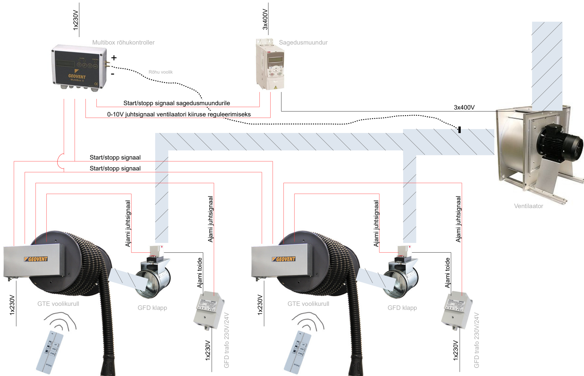
Põhimõtteline ühendusskeem – GTE voolikurullid + ventilaator + röhukontroller + sagedusmuundur + GFD sulgklapid
